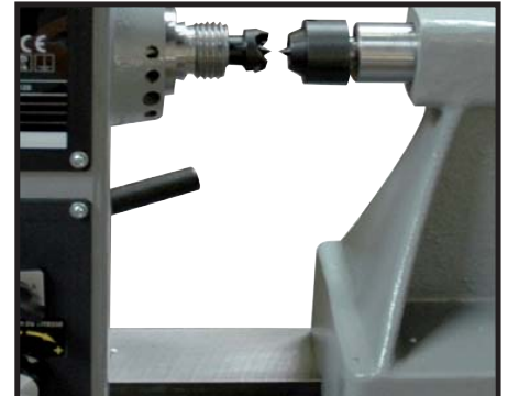
∅ au dessus du banc 460 mm Swing over Bed: 460mm
