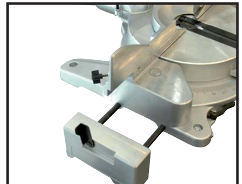
Guide de coupe extensible et rallonges de table Extension cutting guide and extension table
