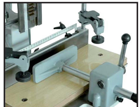
2 presseurs verticaux à serrage rapide et 1 presseur horizontal coulissant 2 vertical vise with quick clamp and 1 horizontal vise
